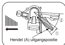
Omschakelen van een klein naar een groter tandwiel (hendel A)
