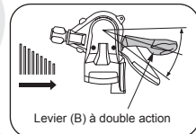
Levier (B) à double action Passage d'une grande couronne dentée vers une plus petite (levier B)
