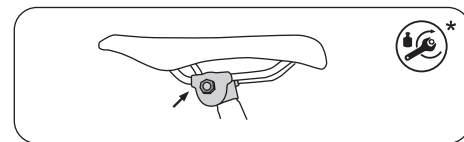
Bevestiging met zadelstrop
