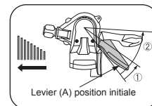
Lever (A) position initiale Passage d'une petite couronne dentée vers une plus grande (levier A)
